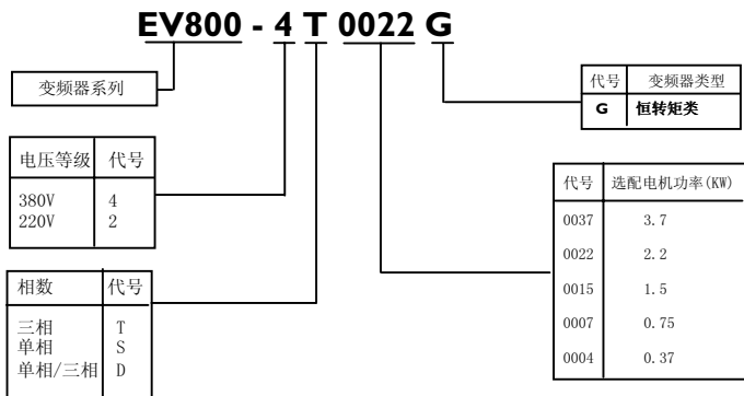
图 2-1a EV800 变频器型号
