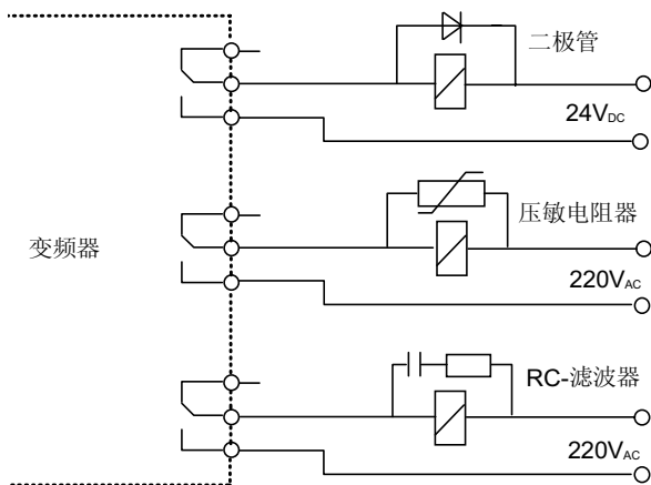
图 3-4 继电器、接触器及电磁制动器要求
