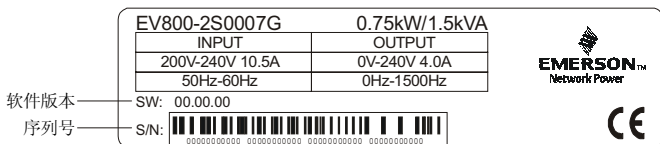
图 2-1b EV800 变频器铭牌
