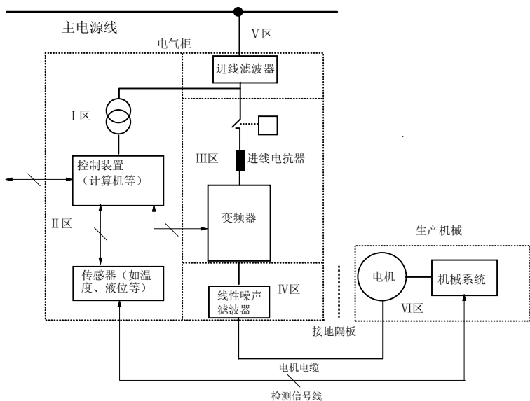
图 3-2 变频器 EMC 安装推荐区域划分示意图
