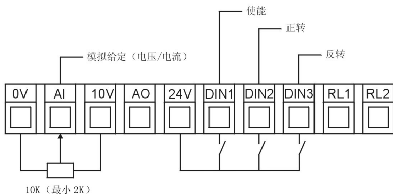
图 5-1 必需的最少控制端子连线
