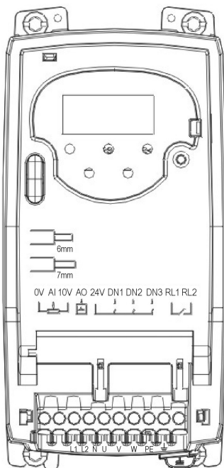
图 3-5 变频器上的各部件（以 SIZE-A 型为例）
