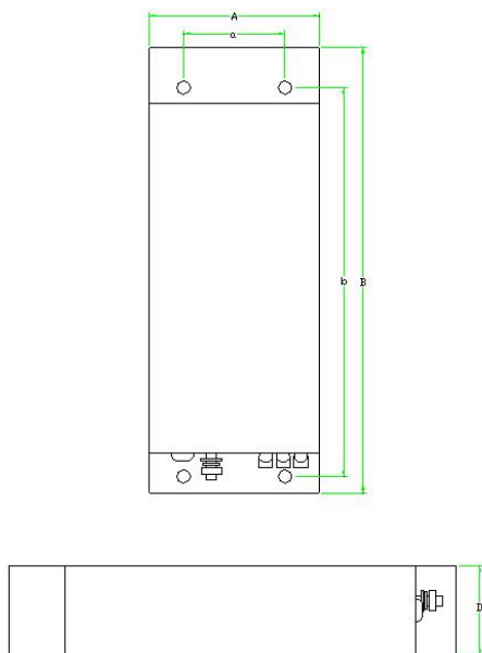
附图 4 EMI 滤波器尺寸图
