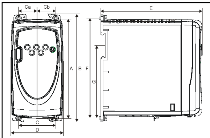
图 2-2 EV800 变频器外形图
